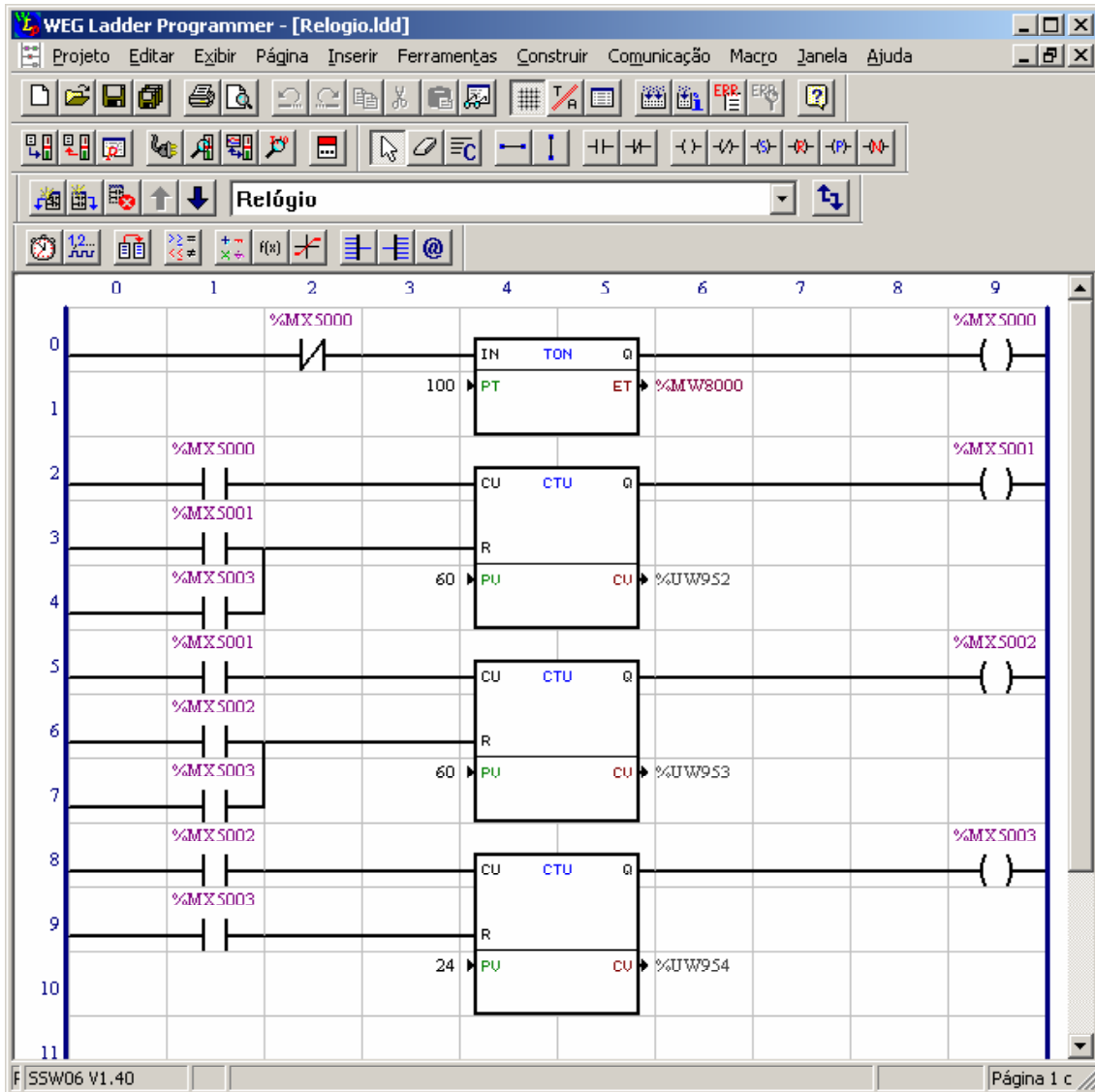
Figura 2.1 - Exemplo de um SoftPLC no software de edição WLP
