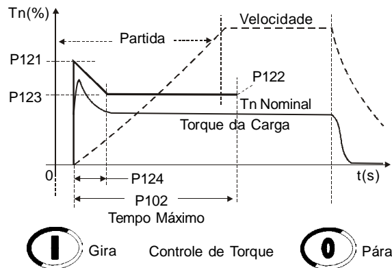
Figura 7.12 - Partida com controle de torque quadrático, 3 pontos, carga inicial mais alta
