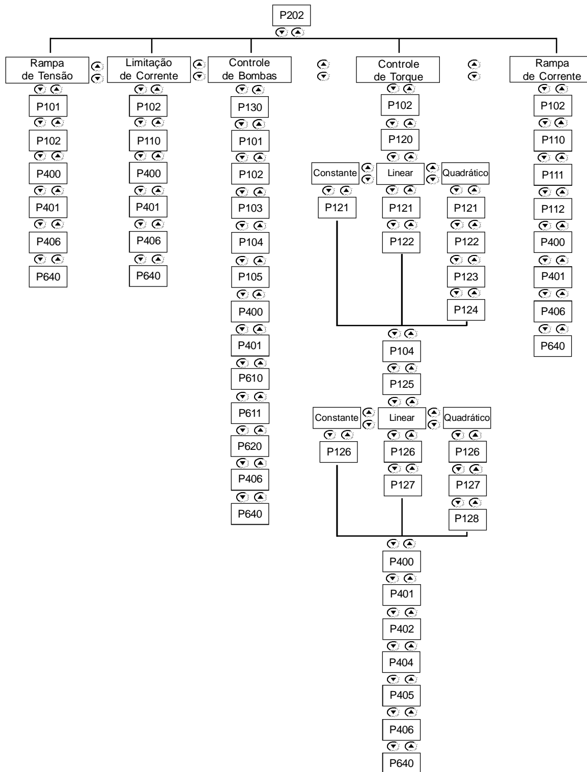
Figura 6.10 - Seqüência de parâmetros conforme o tipo de controle selecionado
