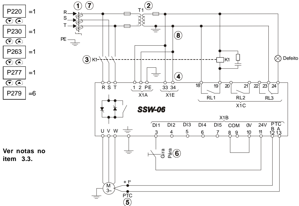
Figura 3.24 - Acionamento sugestivo com comandos por entradas digitais a dois fios
