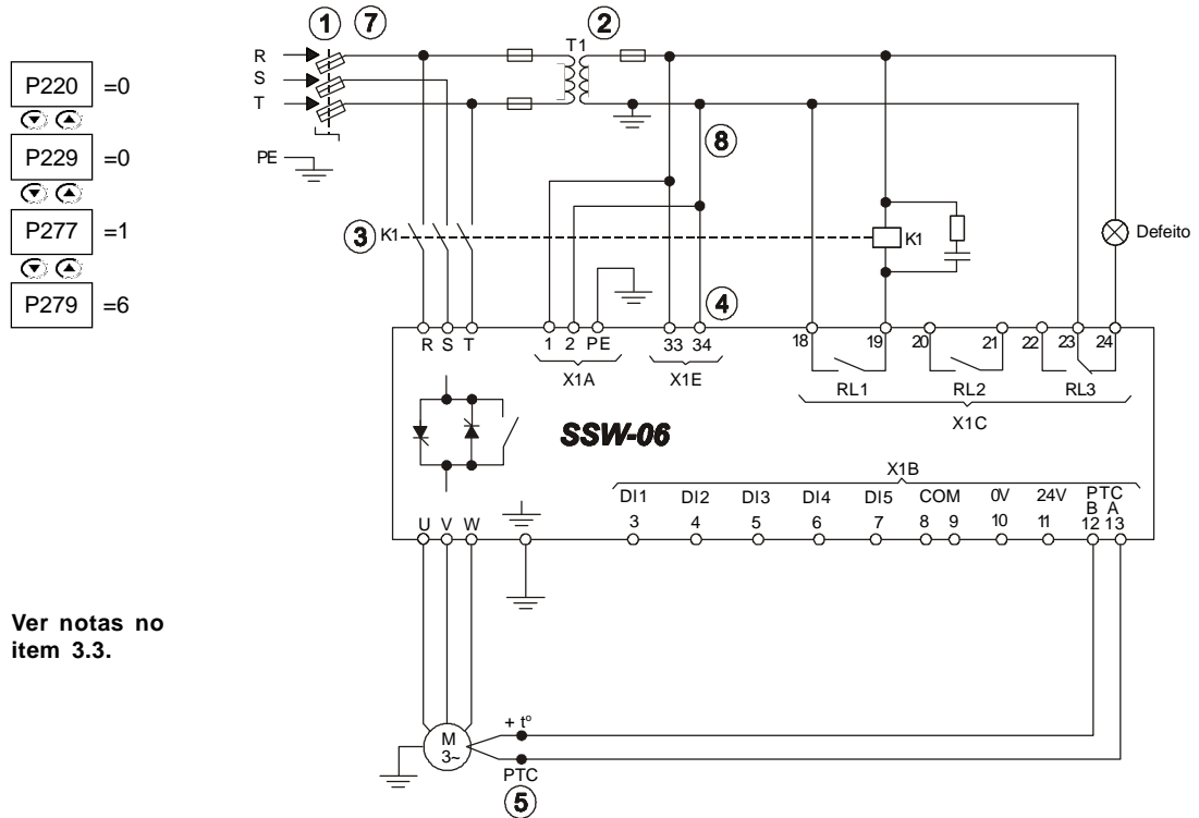
Figura 3.22 - Acionamento sugestivo com comandos por HMI e contator de isolação da potência
