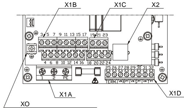
Figura 3.17 - Disposição dos conectores de controle
