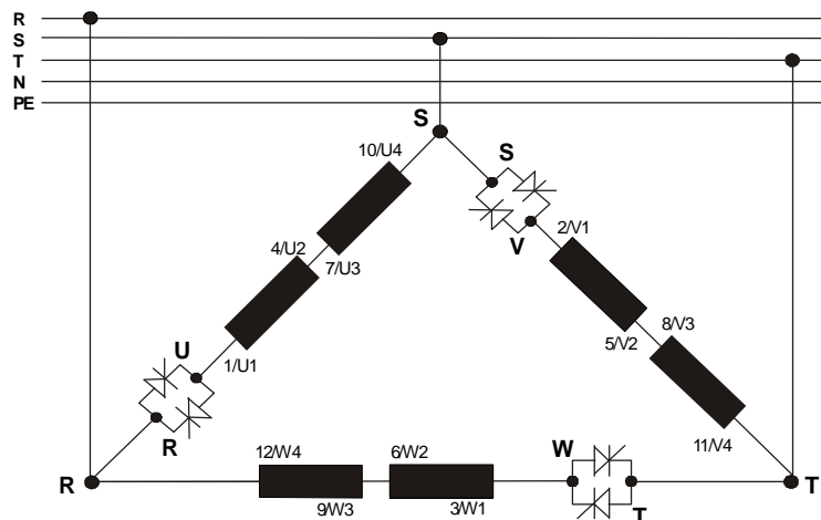
Figura 3.12 - Soft-Starter SSW-06 dentro da ligação delta do motor com motor de duplo delta em série
