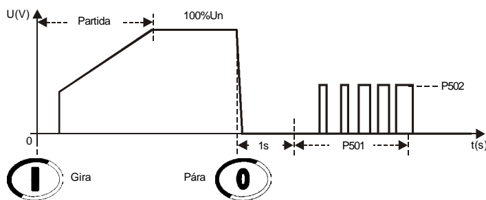
Figura 6.20 - Frenagem Ótima
