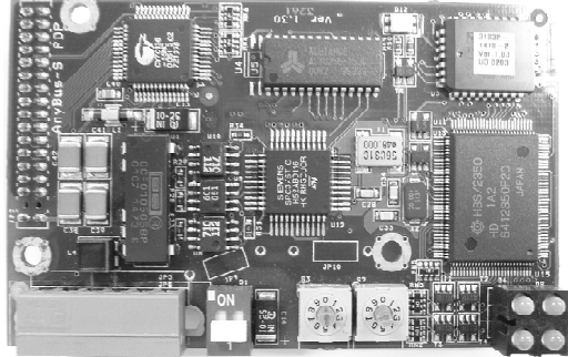
Figura 9.8 - Cartão do Kit opcional Profibus DP
