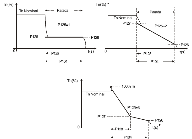
Figura 6.8 - Perfis de torque disponíveis para a parada
