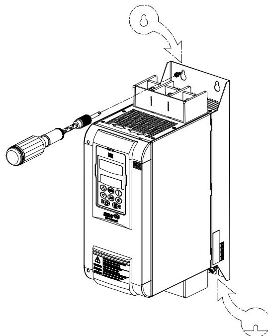
Figura 3.4 - Procedimento de instalação da SSW-06 em superfície
