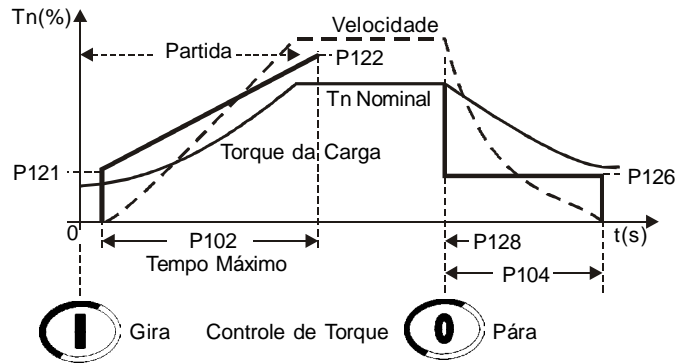
Figura 7.19 - Bomba hidráulica parando com torque constante, 1 ponto
