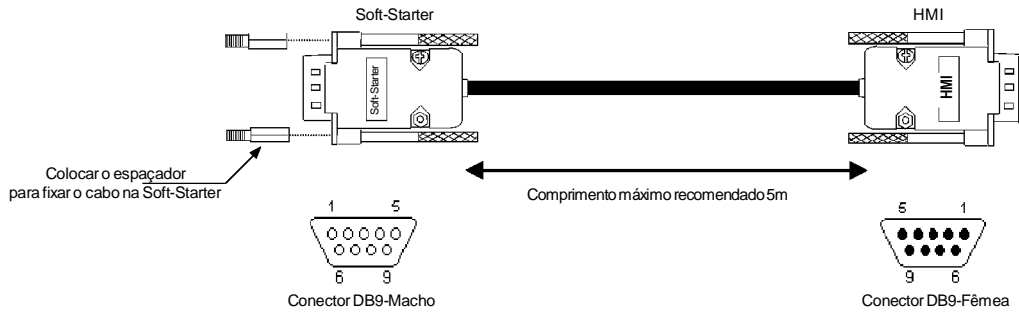
Figura 9.4 - Cabo para uso remoto da HMI
