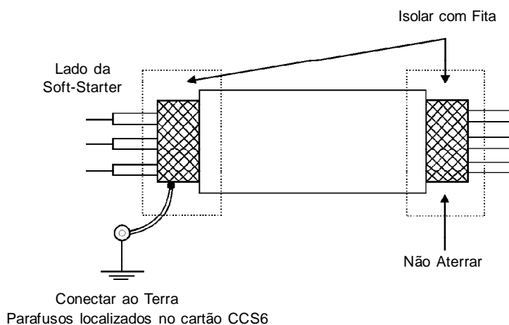
Figura 3.20 - Conexão blindagem
