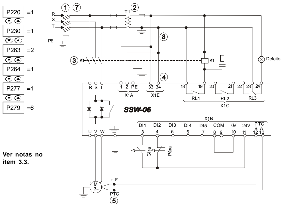
Figura 3.25 - Acionamento sugestivo com comandos por entradas digitais a três fios
