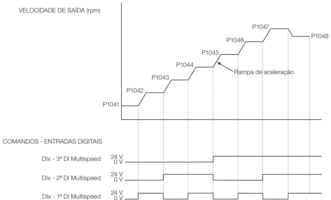
Figura 19.25: Funcionamento da função multispeed
