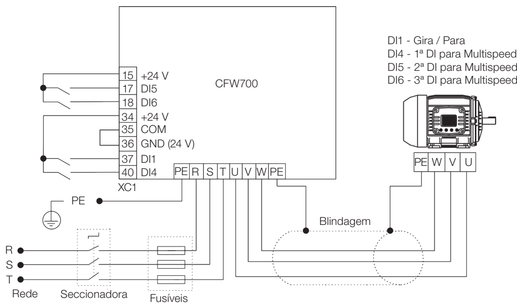
Figura 19.26: Exemplo da função multispeed no CFW700
