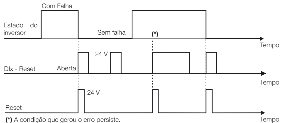
Figura 13.5 (h) a (j) (cont.): Detalhes sobre funcionamento das funções das entradas digitais
