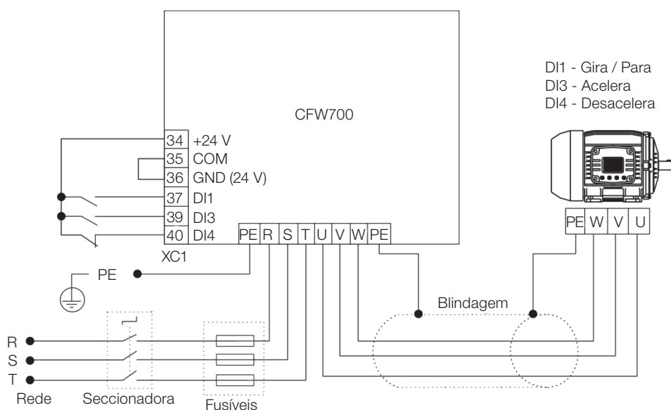
Figura 19.29: Exemplo da função potenciômetro eletrônico no CFW700
