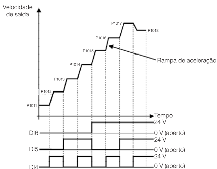
Figura 19.9: Funcionamento da aplicação multispeed
