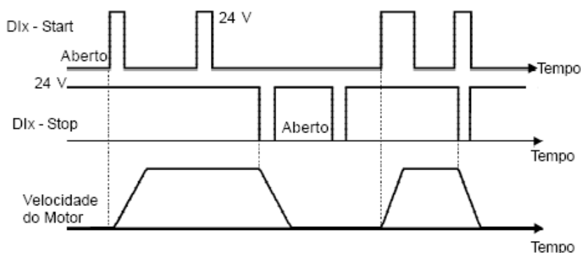
Figura 19.12: Funcionamento da Aplicação Comando a Três Fios (Start / Stop)
