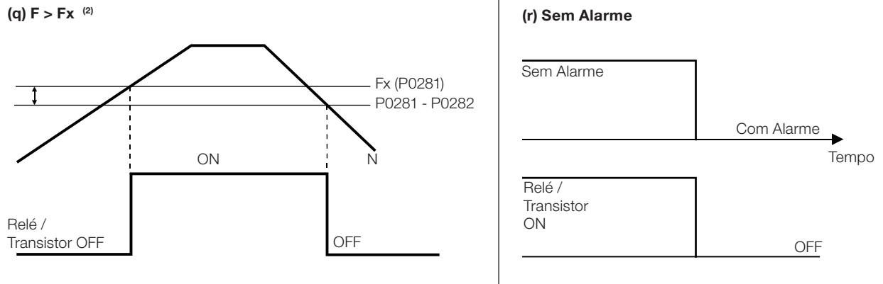
Figura 13.6 (q) e (r) (cont.): Detalhes do funcionamento das funções das saídas digitais e a relé
