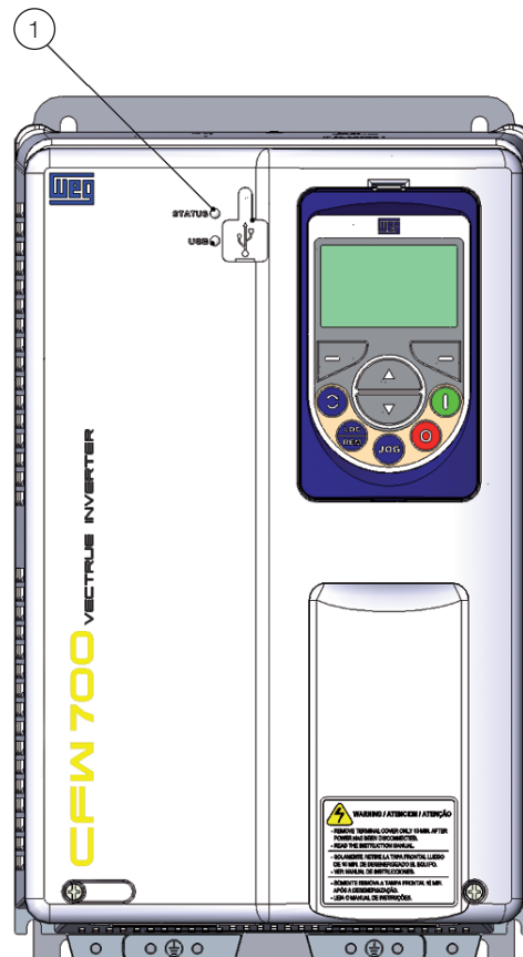
Figura 3.3: LEDs
