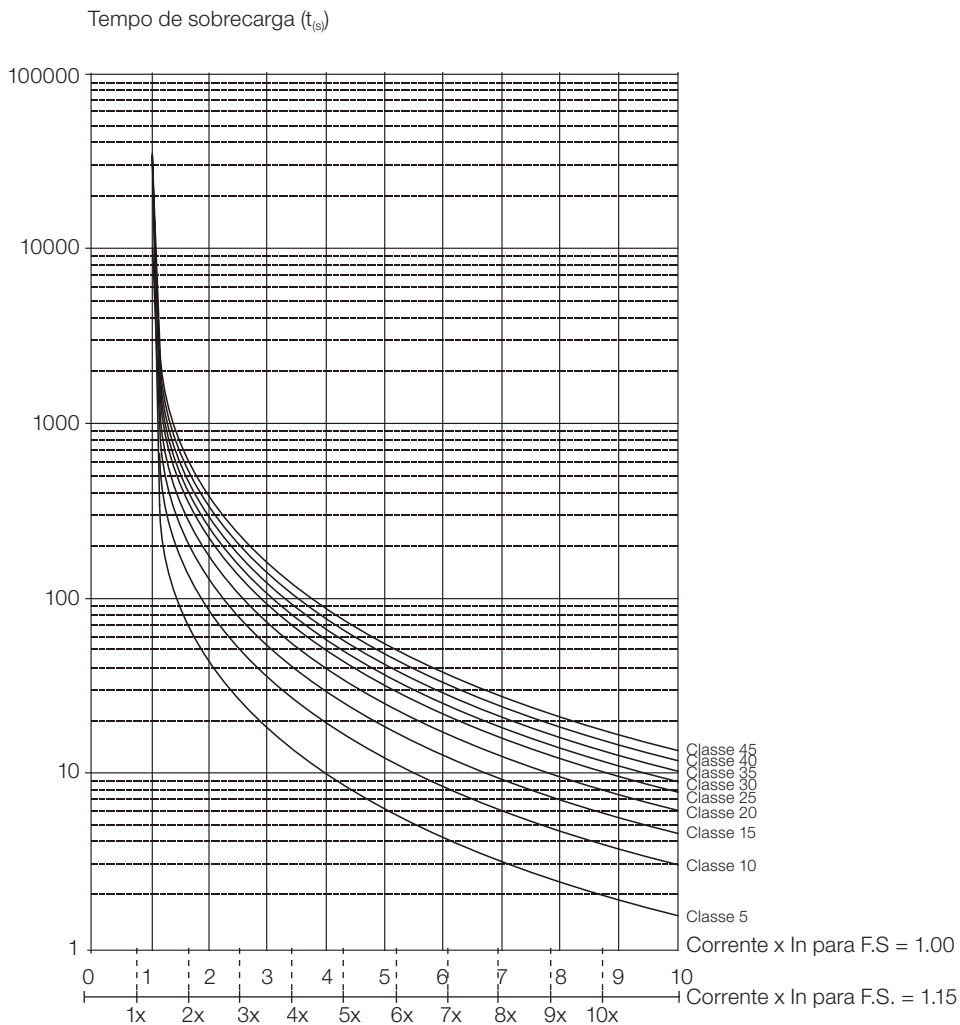
Figura 15.3 (a): Curvas de sobrecarga com o motor a frio para cargas do tipo HD e ND
