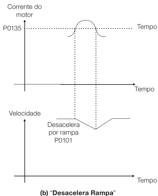
Figura 9.8: Modos de atuação da limitação de corrente via P0135
