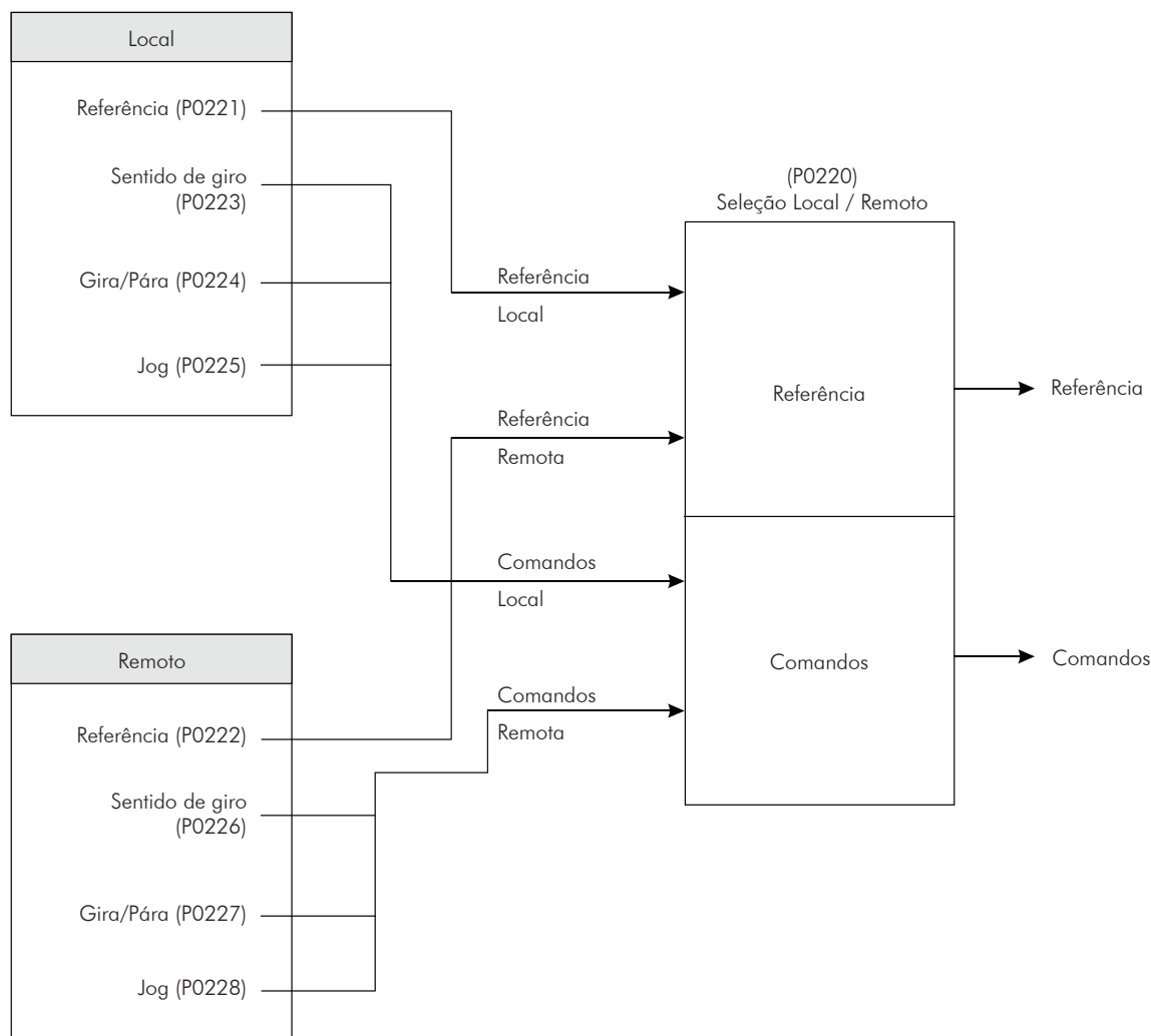
Figura 13.9 - Blocodograma Situação Local / Remoto
