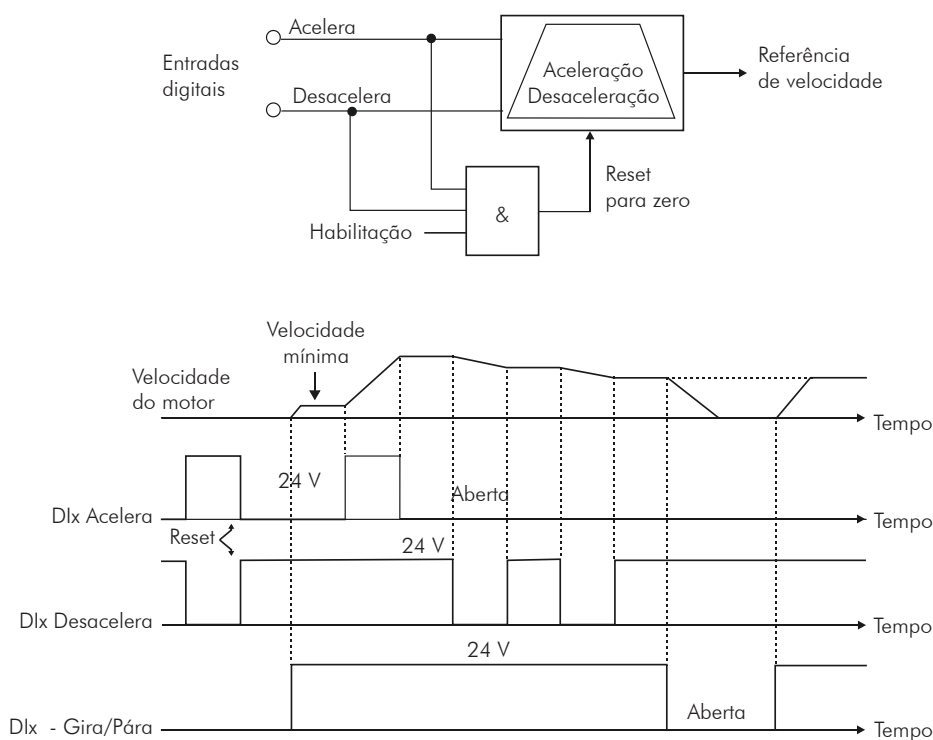
Figura 13.6 (cont.) (k) a (m) - Detalhes sobre funcionamento das funções das Entradas digitais
