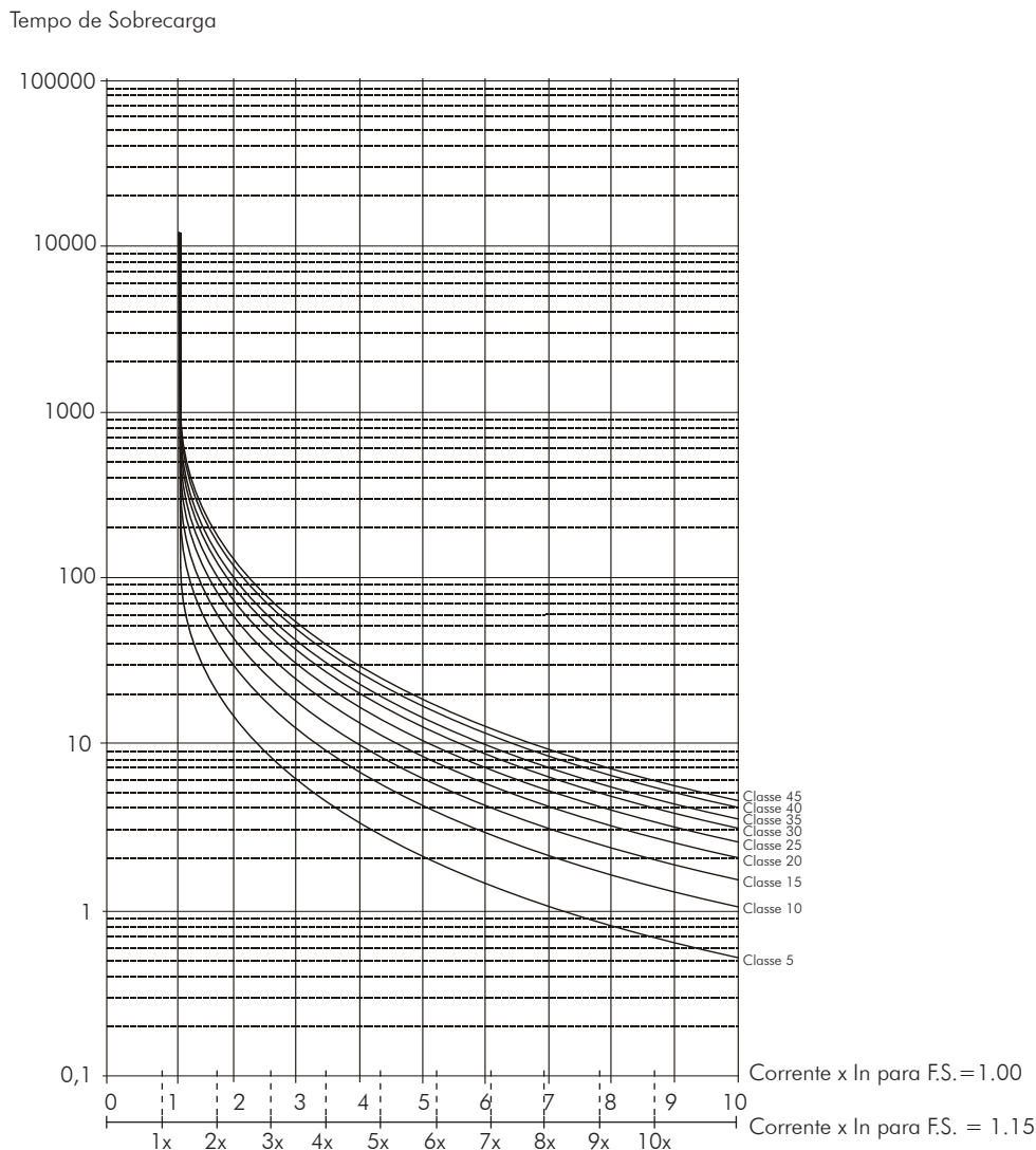
Figura 15.3 (b) - Curvas de sobrecarga com o motor a quente para cargas do tipo HD e ND
