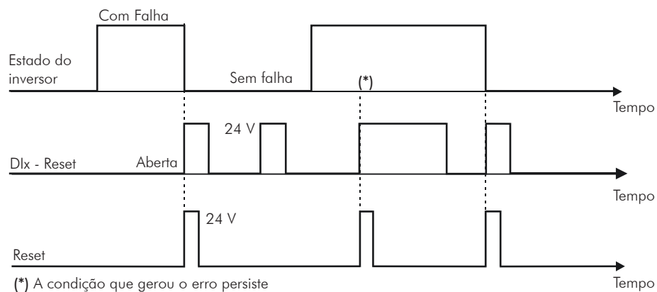
Figura 13.6 (cont.) (h) a (j) - Detalhes sobre funcionamento das funções das entradas digitais
