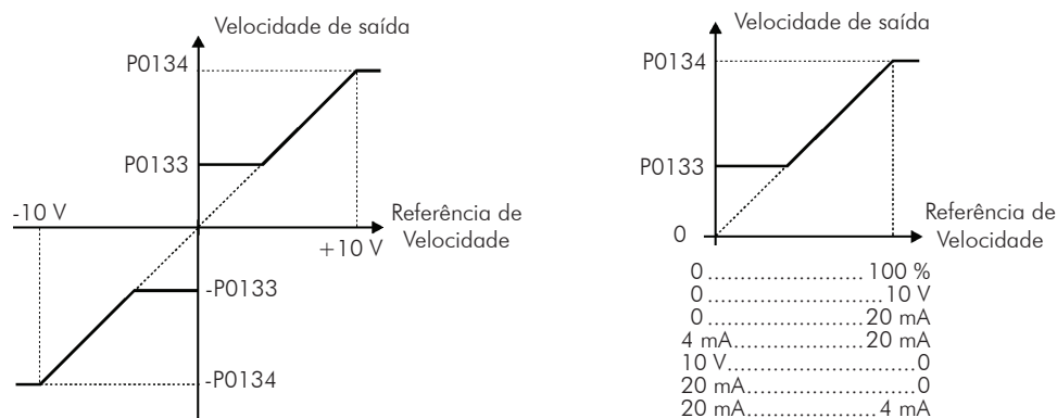
Figura 12.3 (b) - Limites de velocidade considerando "Zona Morta" ativa (P0230=1)
