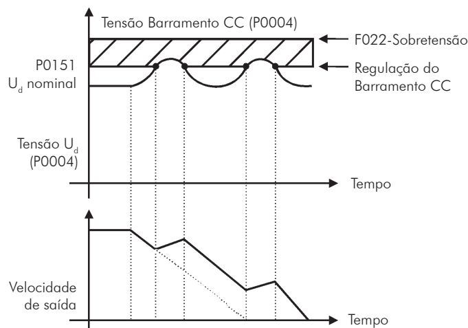
Figura 9.13 - Gráfico exemplo de atuação da limitação da tensão do barramento CC com a função Acelera Rampa
