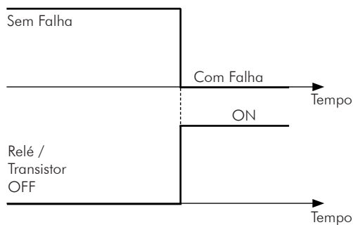
Figura 13.7 (cont.) (e) a (k) - Detalhes do funcionamento das funções das saídas digitais e a relé
