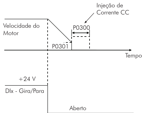
Figura 12.11 (cont.) (b) - Atuação da frenagem CC no bloqueio por rampa (via desabilita rampa)
