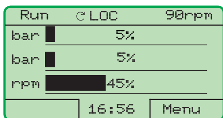
Figura 20.4 - Exemplo da HMI no modo monitoração para a função Regulador PID
