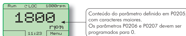
Figura 5.6 - Exemplo de tela no Modo Monitoração com P0205 em caracteres maiores
