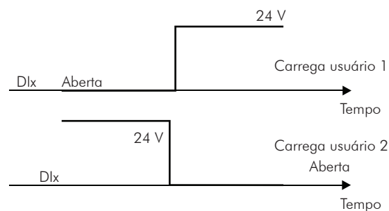
Figura 13.6 (a) a (g) - Detalhes sobre funcionamento das funções das entradas digitais
