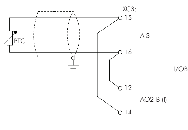
Figura 15.1 (cont.) (d) - Exemplos de conexões do PTC
