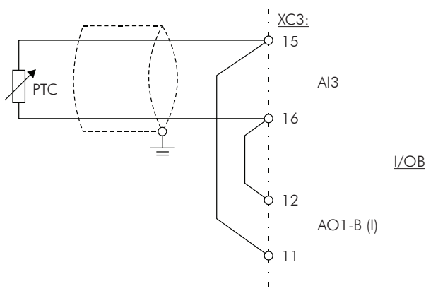
Figura 15.1 (a) a (c) - Exemplos de conexões do PTC
