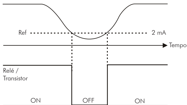
Figura 13.7 (cont.) (e) a (k) - Detalhes do funcionamento das funções das saídas digitais e a relé
