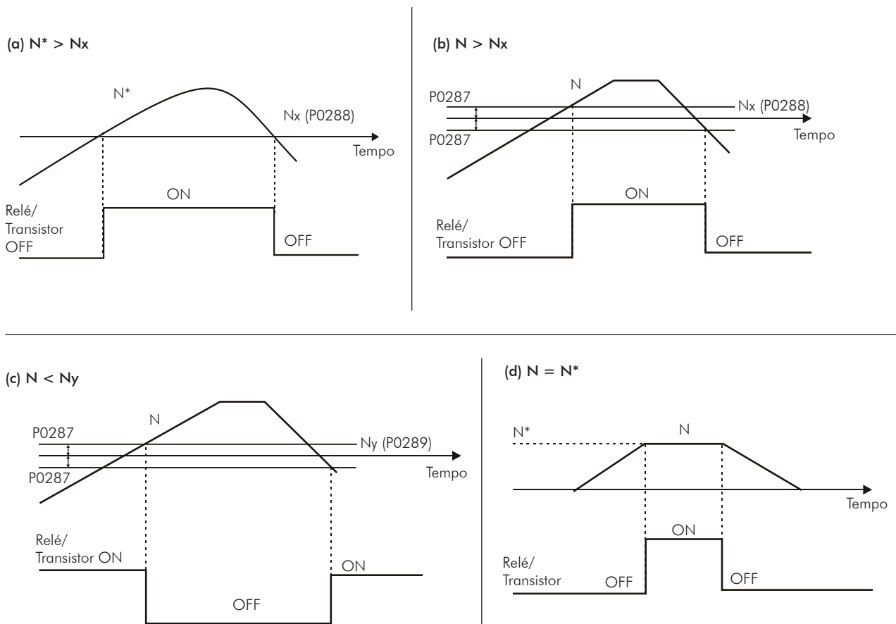
Figura 13.7 (a) a (d) - Detalhes do funcionamento das funções das saídas digitais e a relé
