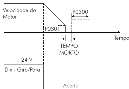
Figura 12.11 (a) - Atuação da frenagem CC no bloqueio por rampa (via desabilita rampa)
