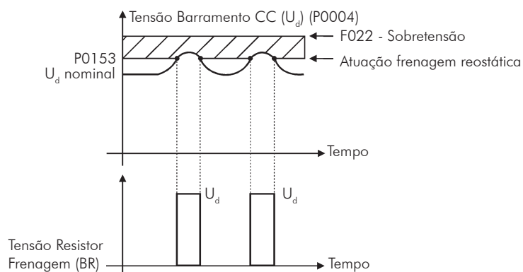
Figura 14.1 - Curva de atuação da Frenagem Reostática
