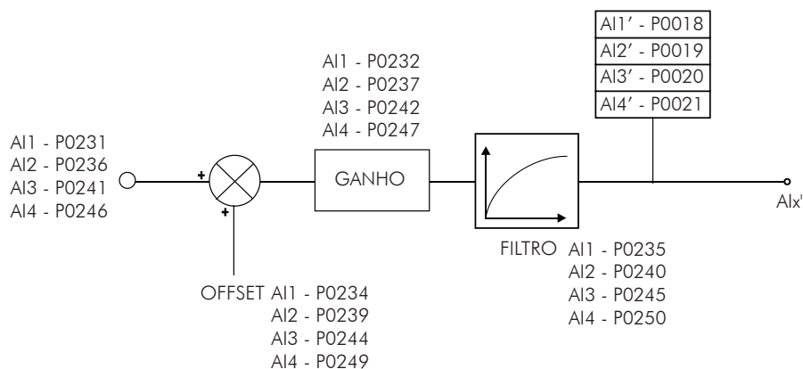
Figura 13.2 - Blocodiagrama das entradas analógicas
