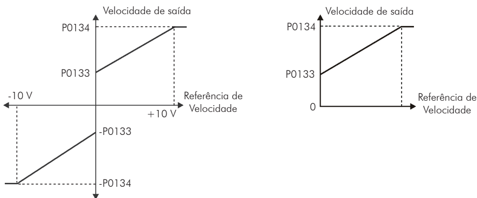
Figura 12.3 (a) - Limites de velocidade considerando "Zona Morta" inativa (P0230=0)
