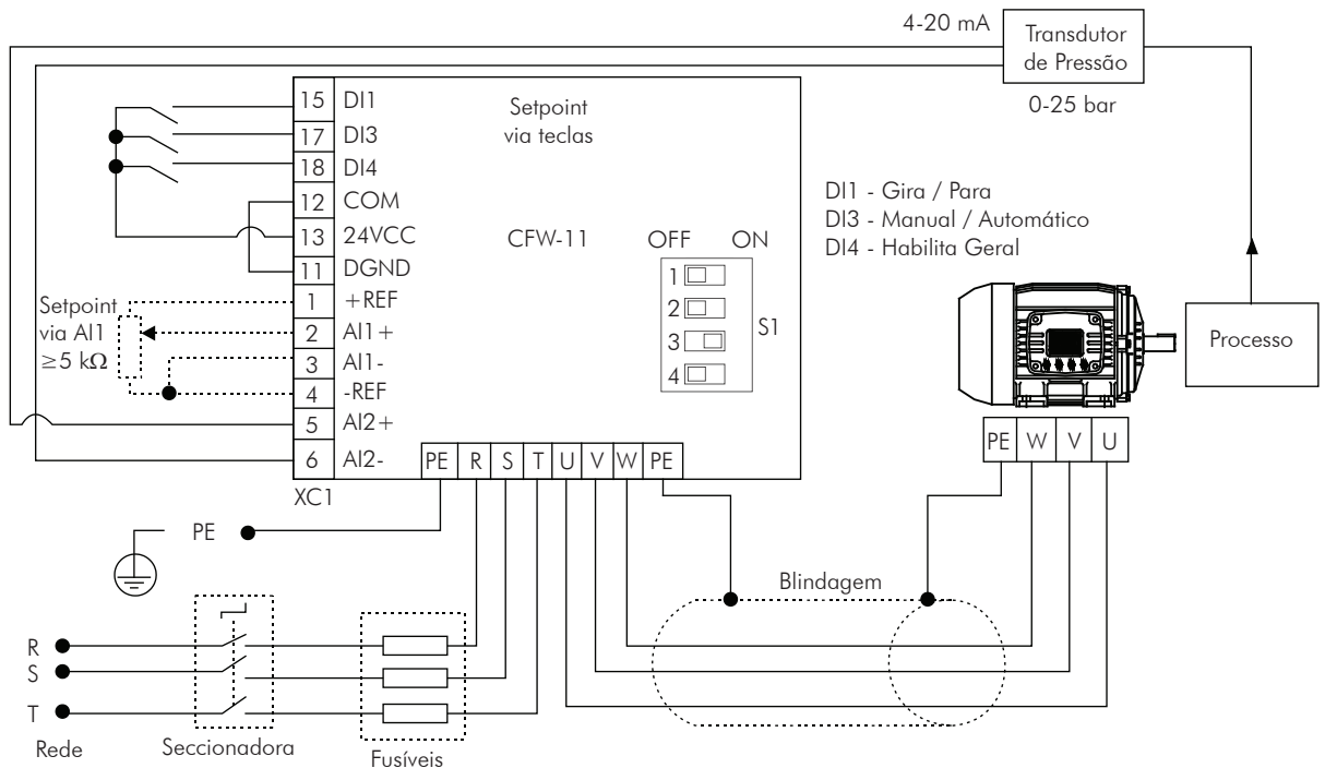
Figura 20.3 - Exemplo de aplicação do CFW-11 como regulador PID
